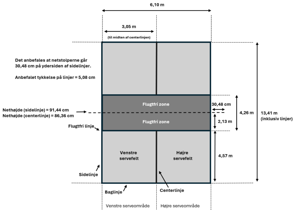
Figur 3 - banens dimensioner.
